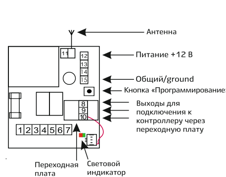
Рис. 1 — Подключение считывателя
