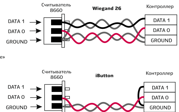
Рис. 1.1 — Подключение переходной платы считывателя к контроллеру
