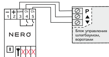
Рис. 2 — Одноканальный режим
