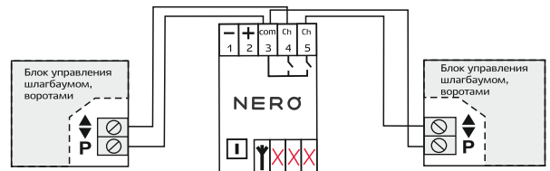
Рис. 3 — Двухканальный режим
